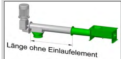
Rohrschnecke RS Z-KG mit Kegelrad-Getriebemotor
