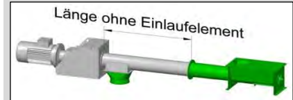
Rohrschnecke RS Z-G mit Getriebemotor
